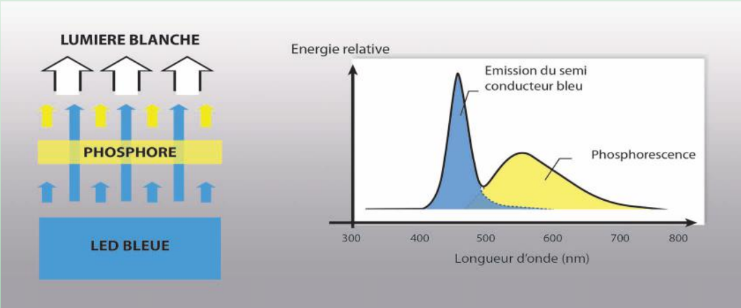
Schéma de conception d'une lampe LED blanche « type » et spectre lumineux associé. Source : Sordello, 2017 [84].
